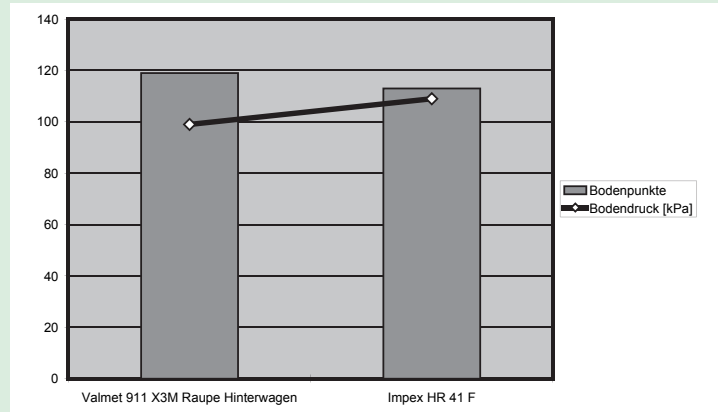
Abb. 4: Vergleich von gemessenem Bodendruck und berechneten Bodenpunkten für 2 Raupenmaschinen
