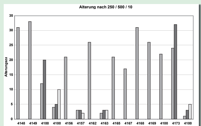
Abb. 3: Alterung nach 250 / 500 / 1000 Stunden
